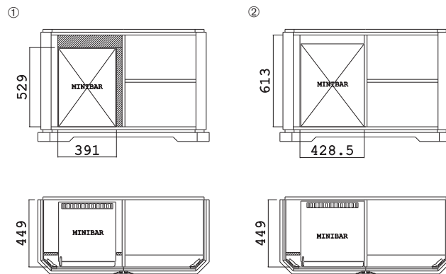
① Innenmaß mit Passleiste / Misura vano con fascia di tamponamento / Measurements with buffer strip
